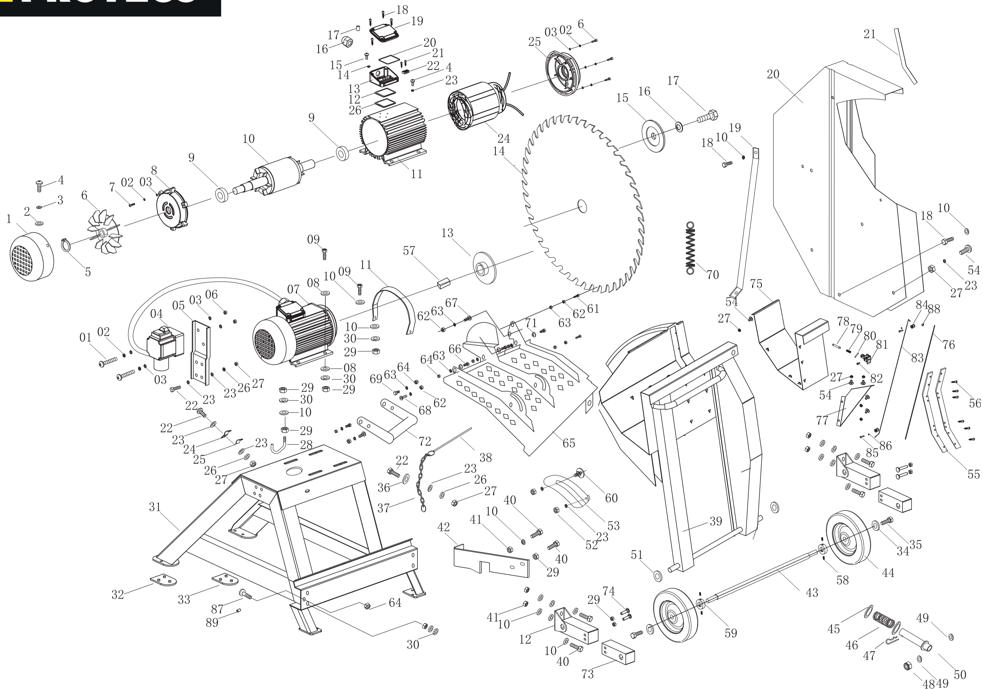
51.01-PH-700 | pila kolébková (cirkulárka) 4kW, 400V, s kotoučem 700mm
