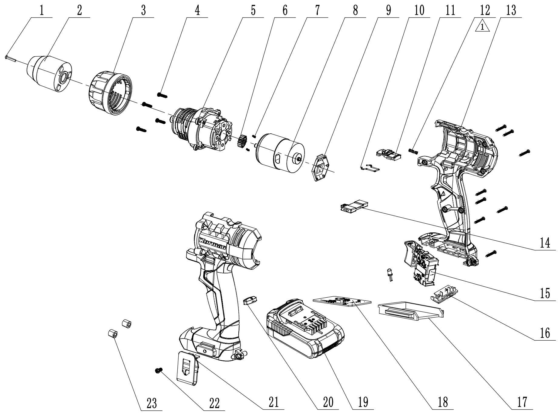
51.10-AV-20-01, 05 | vrtačka akumulátorová 2-13mm 20V, 1 akumulátor
