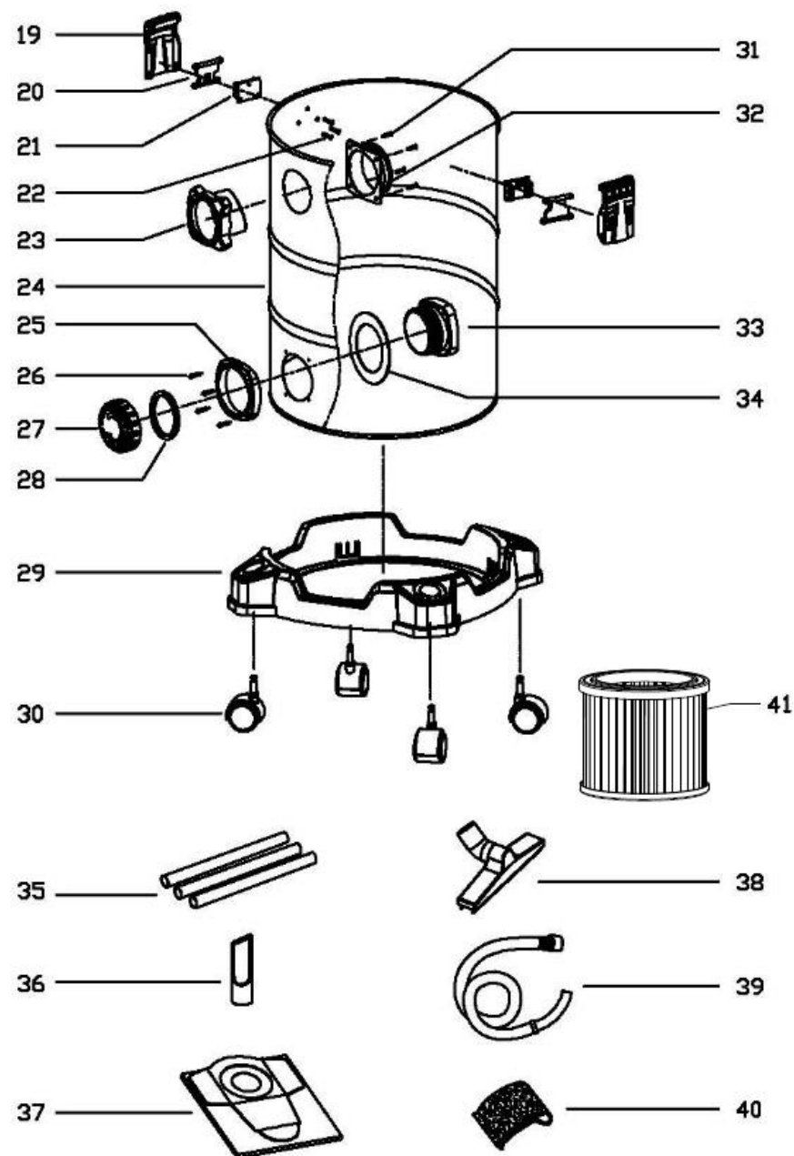
51.14-VP-1200 vysavač průmyslový 1200W s nádobou 20L
