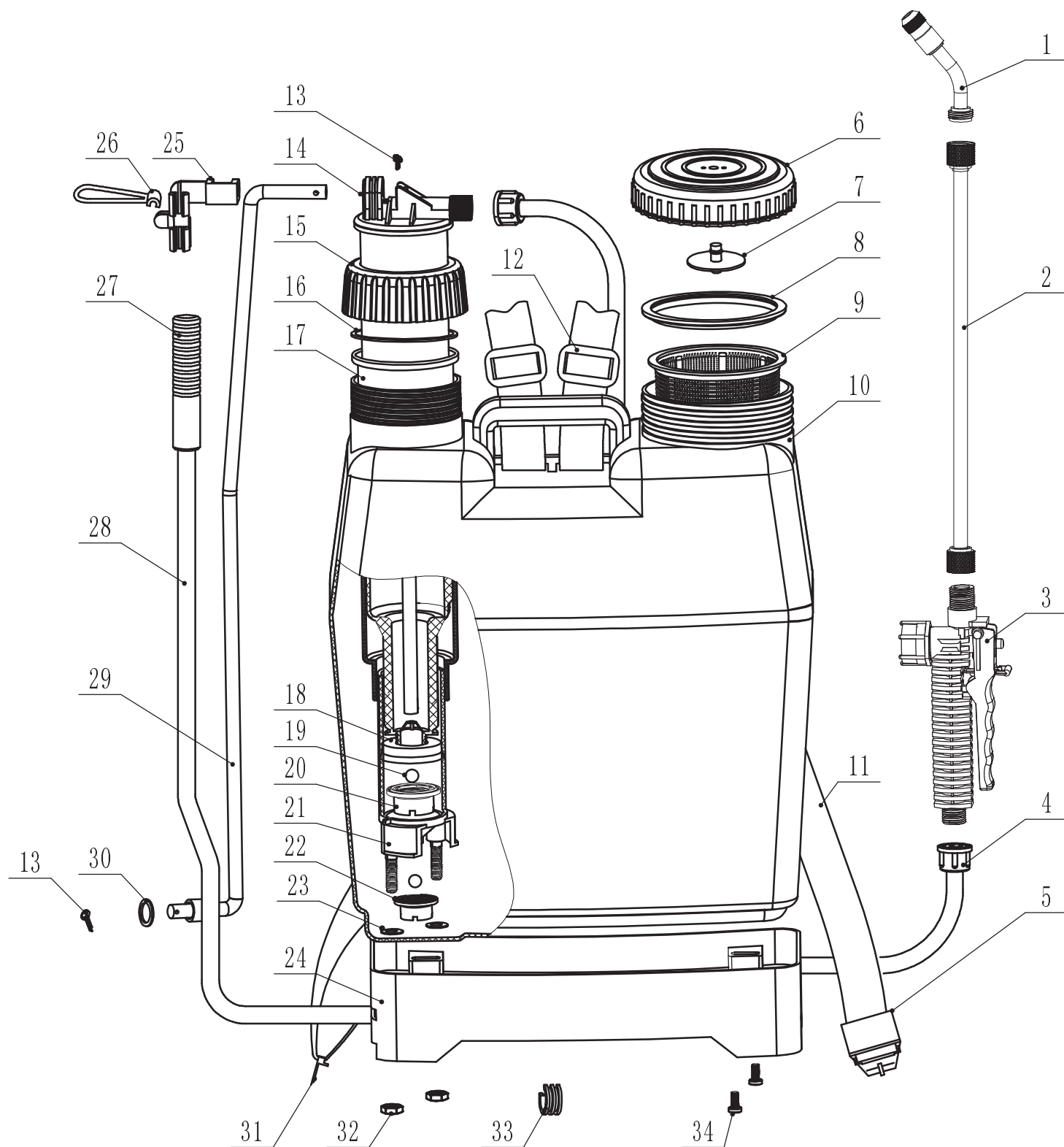
10.80-PT-12 postřikovač 12 L ruční tlakový
